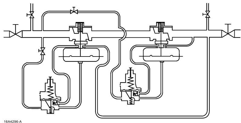
灵活的全开式监控器的安装允许全开式监控器处于上游或下游
