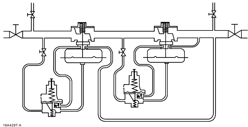
全开式监控器的最小管道的安装要求全开式监控器总是处于上游
